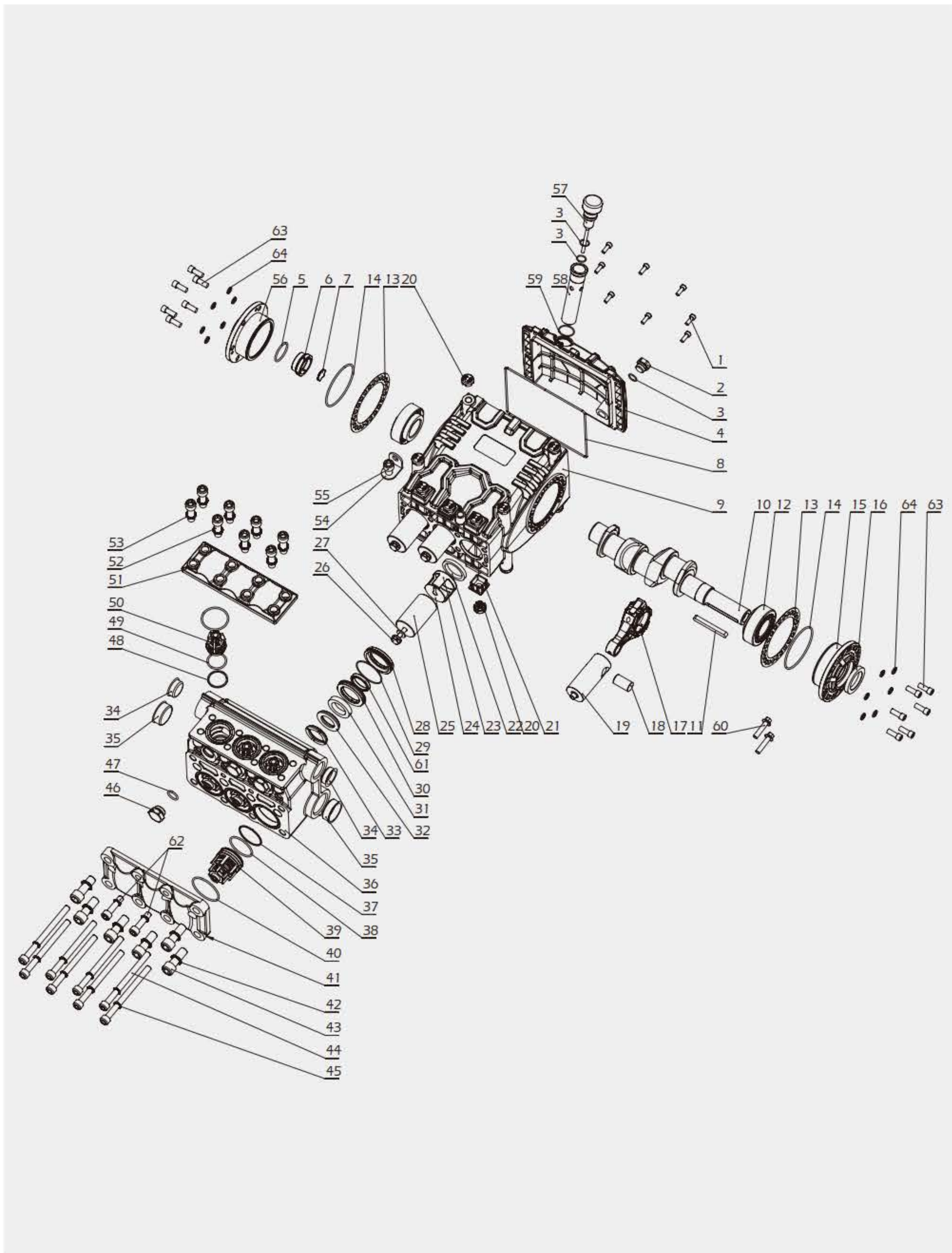
分解图 explosive view
